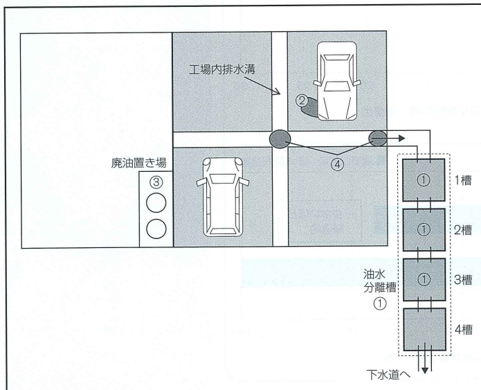
図 工場内でのオイル吸着材使用例
