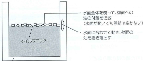
油水分離槽
